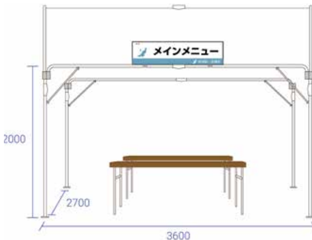
〈テント立面図〉
