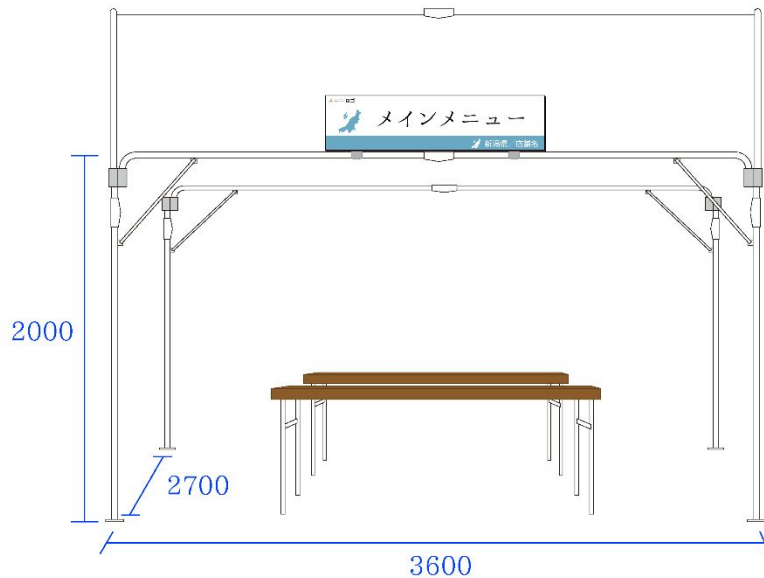
《テント立面図》
